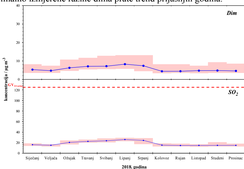
Slika 2. Kretanje srednjih dnevnih koncentracija sumporova dioksida i dima na području Općine Raša u 2018. godini
