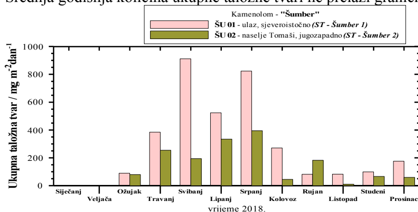
Slika 8. Kretanje mjesečnih količina ukupnih taložnih tvari za razdoblje u 2018. godini
