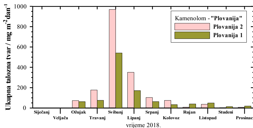
Slika 6. Kretanje mjesečnih količina ukupnih taložnih tvari za razdoblje u 2018. godini
