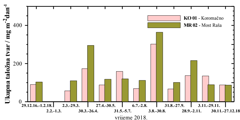
Slika 5. Kretanje mjesečnih količina ukupnih taložnih tvari u 2018. godini
