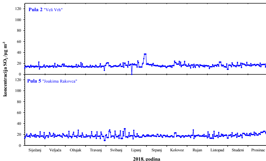
Slika 1. Kretanje srednjih dnevnih koncentracija sumporova dioksida na području Grada Pule u 2018. godini
