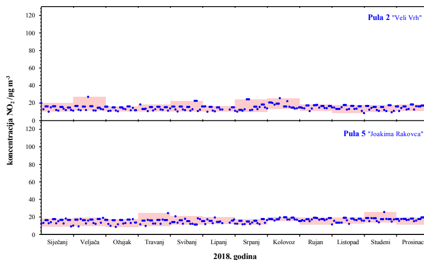
Slika 3. Kretanje srednjih dnevnih koncentracija dušikova dioksida na području Grada Pule u 2018. godini
