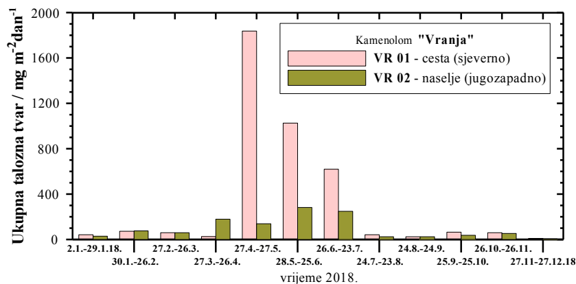
Slika 7. Kretanje mjesečnih količina ukupnih taložnih tvari za razdoblje u 2018. godini
