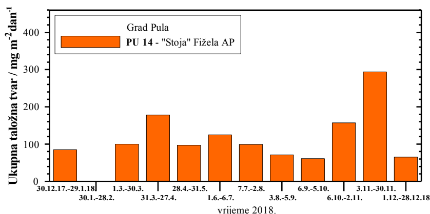
Slika 4. Kretanje mjesečnih količina ukupnih taložnih tvari za razdoblje u 2018. godini
