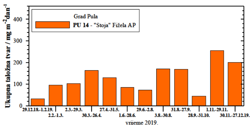
Slika 4. Kretanje mjesečnih količina ukupnih taložnih tvari za razdoblje u 2019. godini
