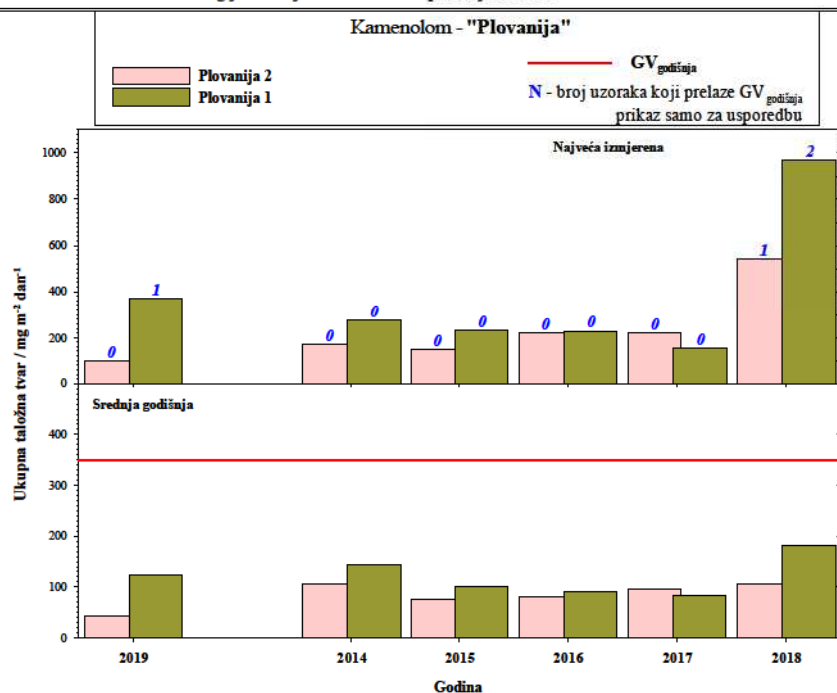
Slika 17. Usporedba rezultata mjerenja ukupne taložne tvari sa kriterijima za vrednovanje kvalitete zraka na mjernim postajama kamenoloma Plovanija
