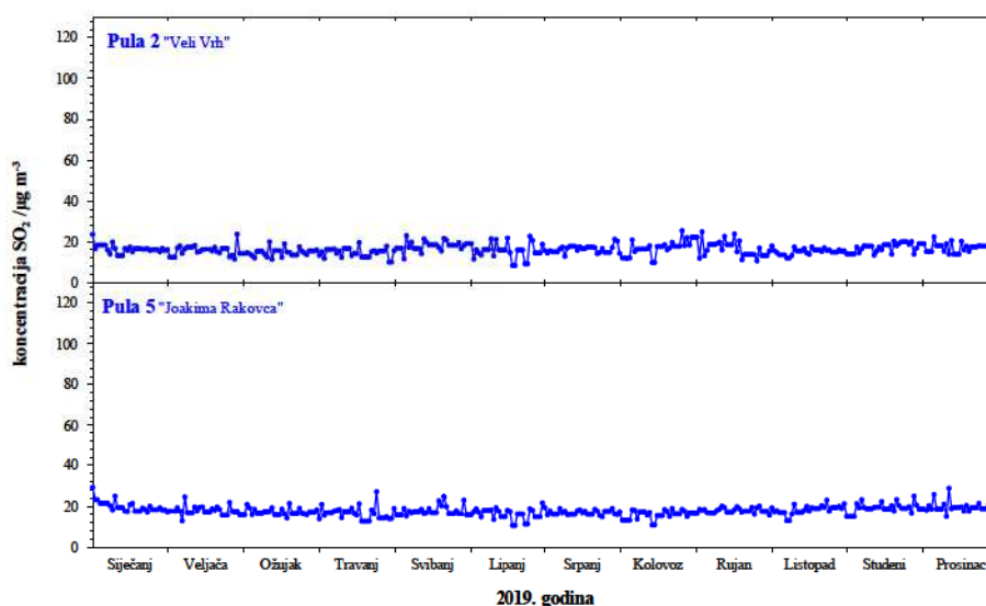
Slika 1. Kretanje srednjih dnevnih koncentracija sumporova dioksida na području Grada Pule u 2019. godini
