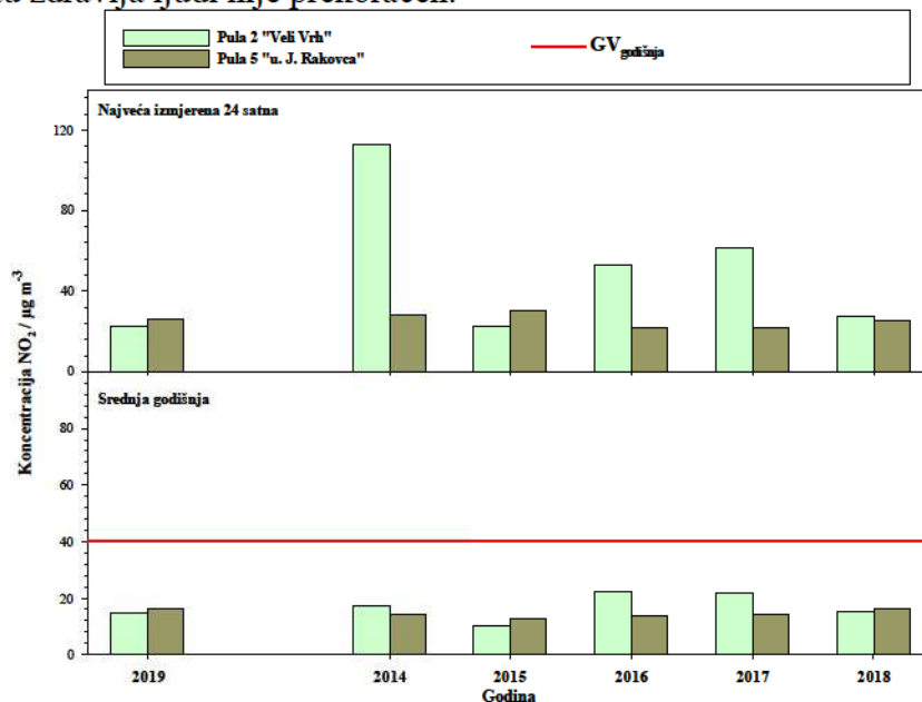
Slika 11. Usporedba rezultata mjerenja dušikova dioksida sa kriterijima za vrednovanje kvalitete zraka na području Grada Pule
