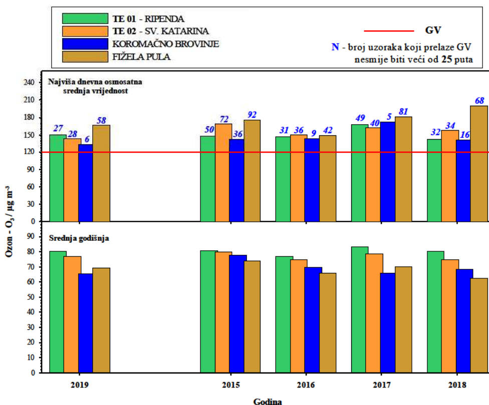
Slika 13. Usporedba rezultata mjerenja ozona sa kriterijima za vrednovanje kvalitete zraka mjerenih na automatskim postajama
