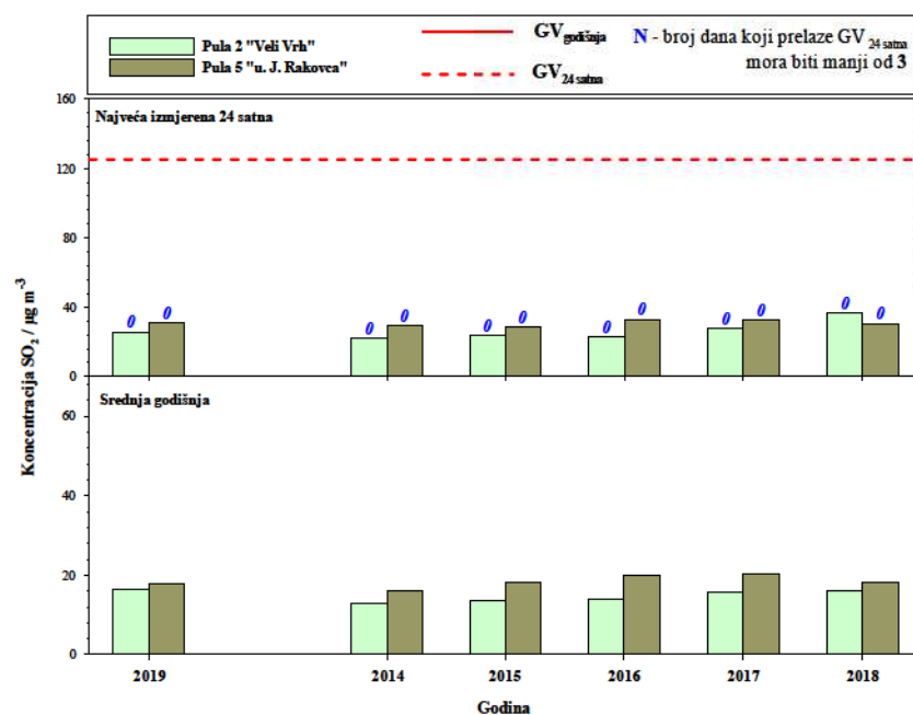
Slika 8. Usporedba rezultata mjerenja sumporova dioksida sa kriterijima za vrednovanje kvalitete zraka na području Grada Pule
