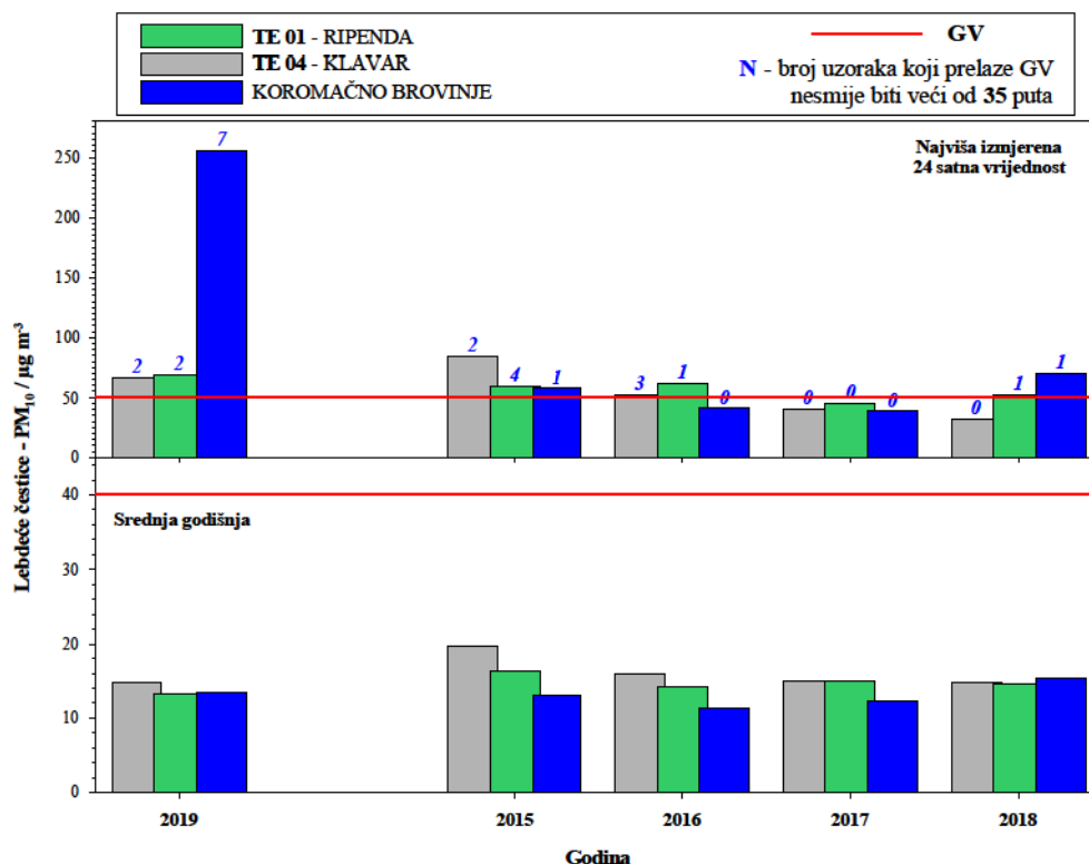
Slika 14. Usporedba rezultata mjerenja koncentracija lebdećih čestica sa kriterijima za vrednovanje kvalitete zraka mjerenih na automatskim postajama
