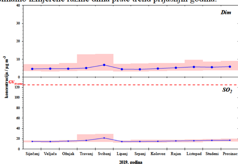
Slika 2. Kretanje srednjih dnevnih koncentracija sumporova dioksida i dima na području Općine Raša u 2019. godini
