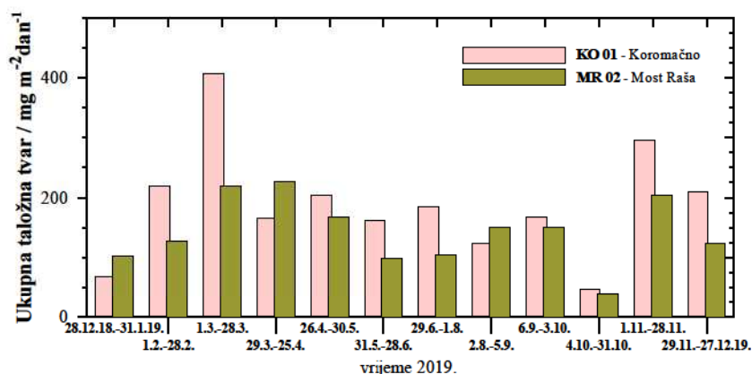
Slika 5. Kretanje mjesečnih količina ukupnih taložnih tvari u 2019. godini
