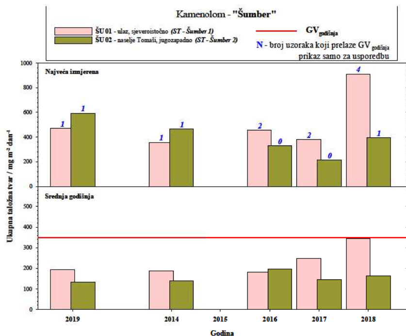
Slika 18. Usporedba rezultata mjerenja ukupne taložne tvari sa kriterijima za vrednovanje kvalitete zraka na mjernim postajama kamenoloma Šumber
