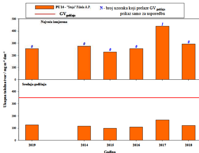
Slika 15. Usporedba rezultata mjerenja ukupne taložne tvari sa kriterijima za vrednovanje kvalitete zraka na mjernoj postaji Grada Pule
