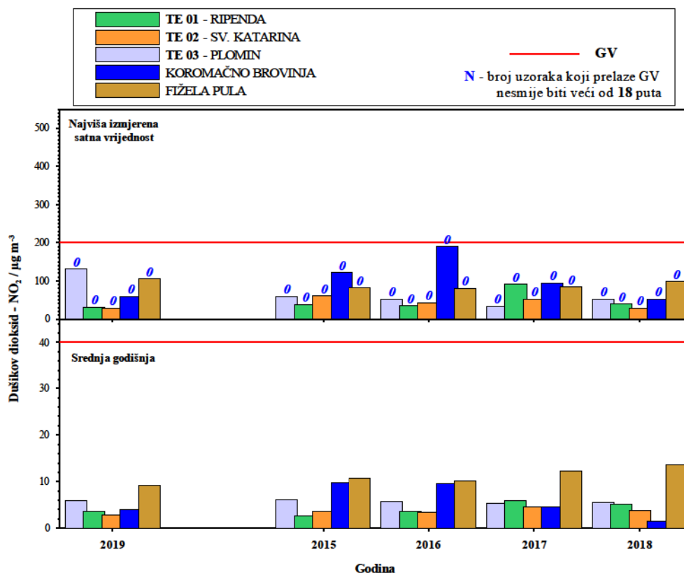
Slika 12. Usporedba rezultata mjerenja dušikova dioksida sa kriterijima za vrednovanje kvalitete zraka mjerenih na automatskim postajama
