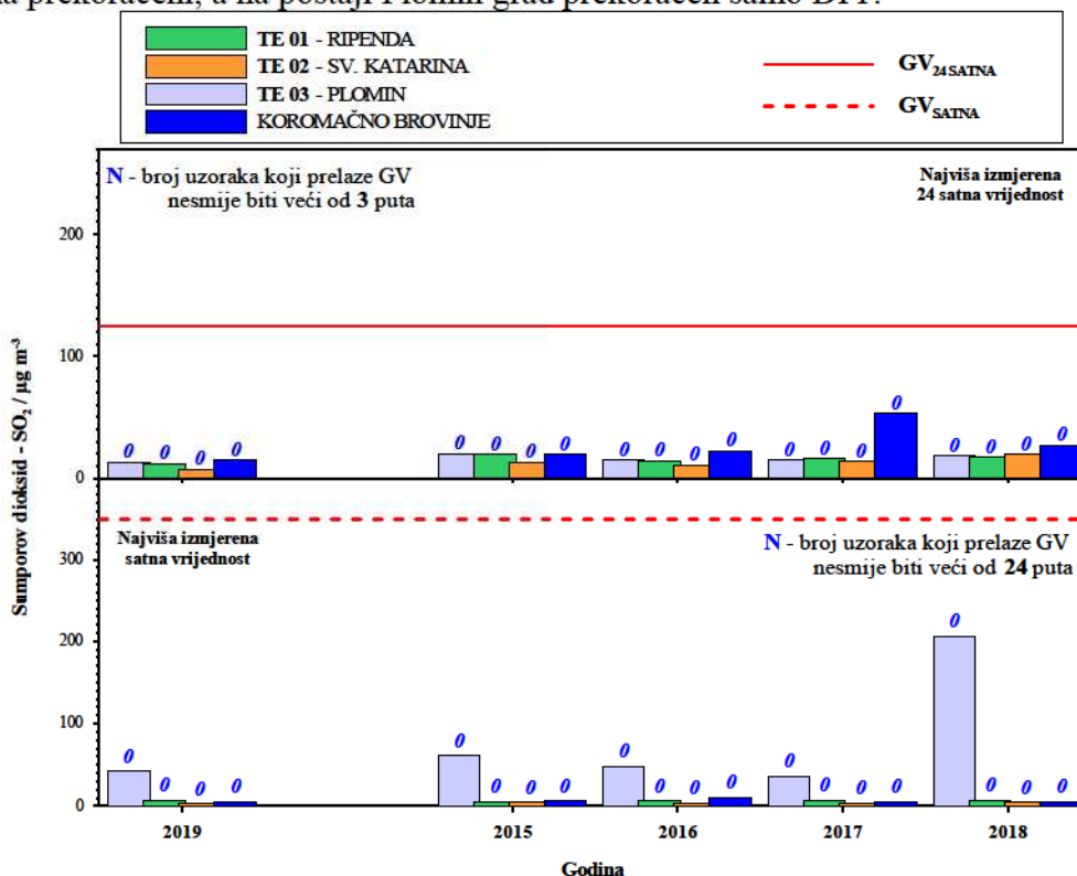
Slika 10. Usporedba rezultata mjerenja sumporova dioksida sa kriterijima za vrednovanje kvalitete zraka mjerenih na automatskim postajama
