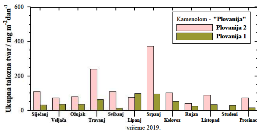
Slika 6. Kretanje mjesečnih količina ukupnih taložnih tvari za razdoblje u 2019. godini
