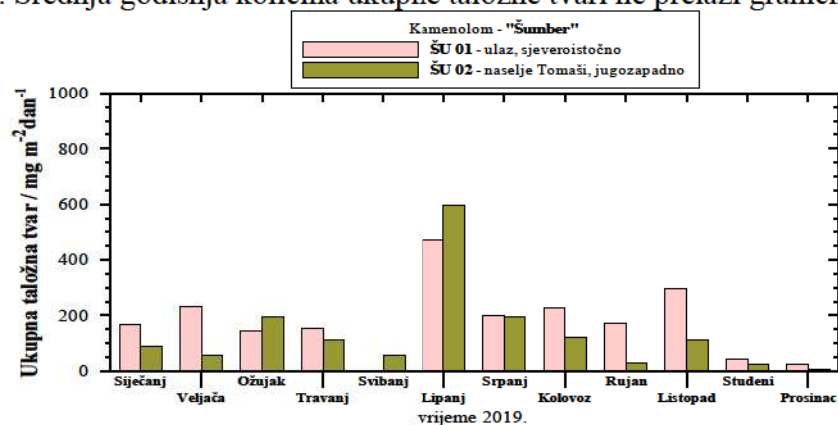
Slika 7. Kretanje mjesečnih količina ukupnih taložnih tvari za razdoblje u 2019. godini
