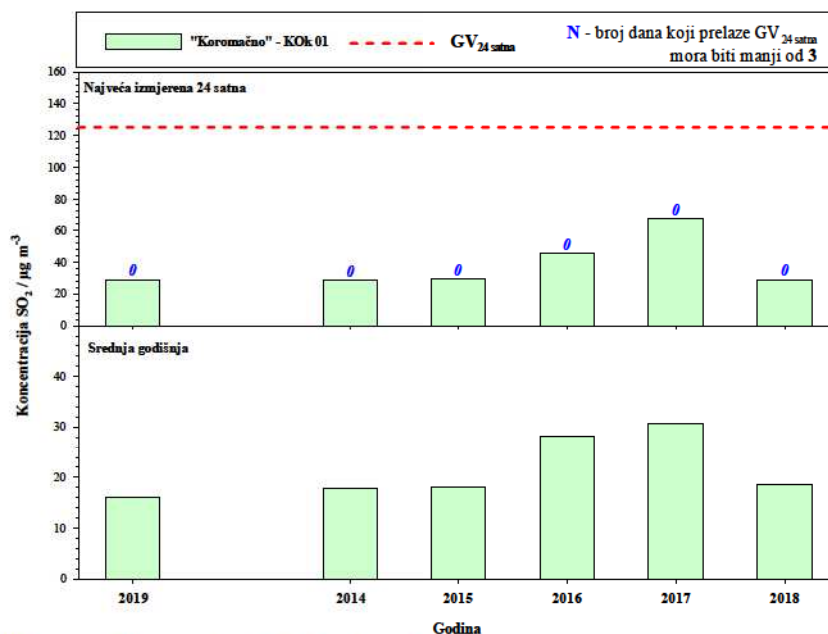
Slika 9. Usporedba rezultata mjerenja sumporova dioksida sa kriterijima za vrednovanje kvalitete zraka na području Općine Raša
