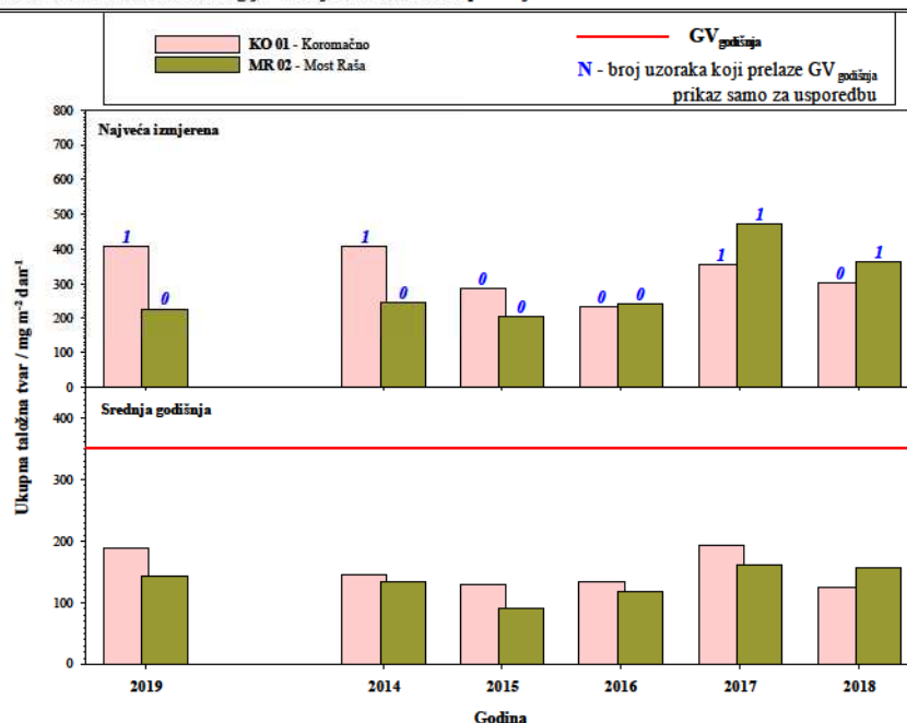
Slika 16. Usporedba rezultata mjerenja ukupne taložne tvari sa kriterijima za vrednovanje kvalitete zraka na području Općine Raša
