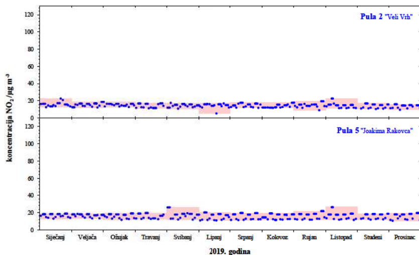
Slika 3. Kretanje srednjih dnevnih koncentracija dušikova dioksida na području Grada Pule u 2019. godini
