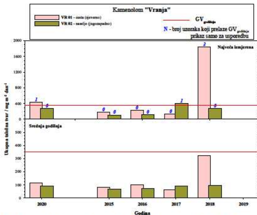
Slika 20. Usporedba rezultata mjerenja ukupne taložne tvari sa kriterijima za
