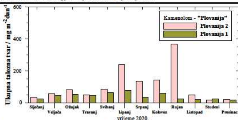
Slika 6. Kretanje mjesečnih količina ukupnih taložnih tvari za razdoblje u 2020. godini
