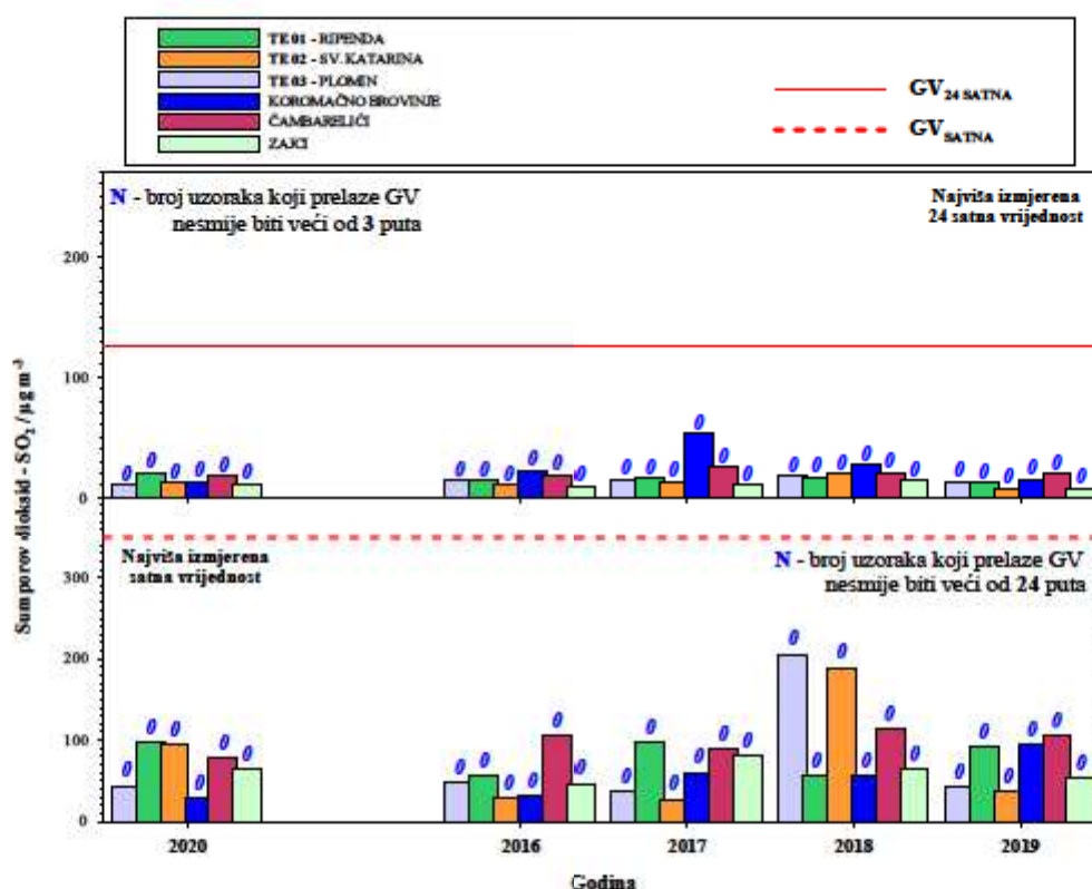
Slika 11. Usporedba rezultata mjerenja sumporova dioksida sa kriterijima za vrednovanje kvalitete zraka mjerenih na automatskim postajama
