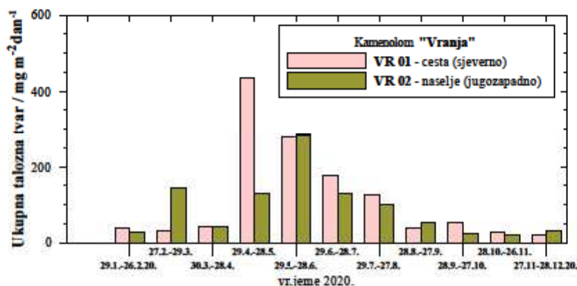
Slika 7. Kretanje mjesečnih količina ukupnih taložnih tvari za razdoblje u 2020. godini
