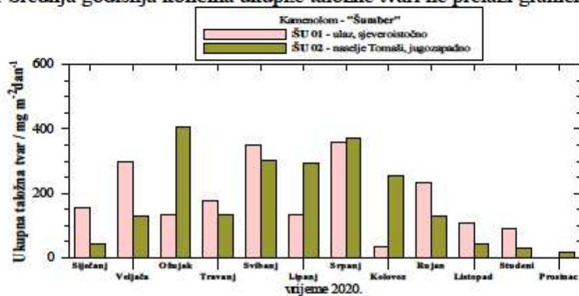
Slika 8. Kretanje mjesečnih količina ukupnih taložnih tvari za razdoblje u 2020. godini
