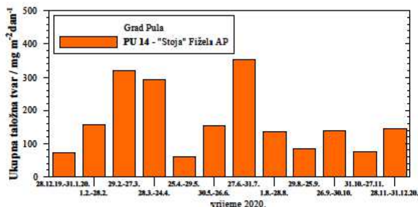
Slika 4. Kretanje mjesečnih količina ukupnih taložnih tvari za razdoblje u 2020. godini
