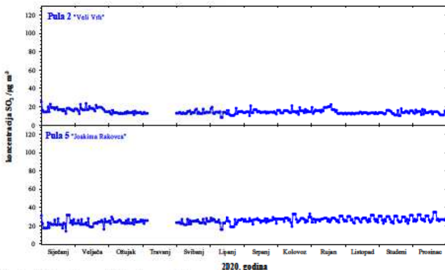
Slika 1. Kretanje srednjih dnevnih koncentracija sumporova dioksida na području Grada Pule u 2020. godini
