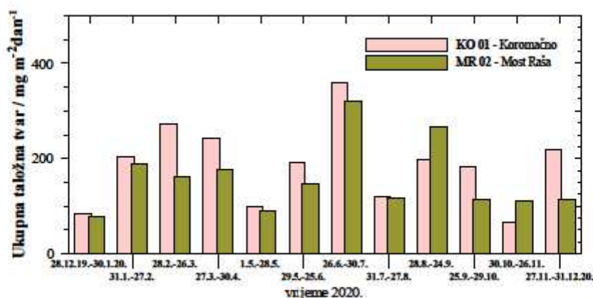
Slika 5. Kretanje mjesečnih količina ukupnih taložnih tvari u 2020. godini
