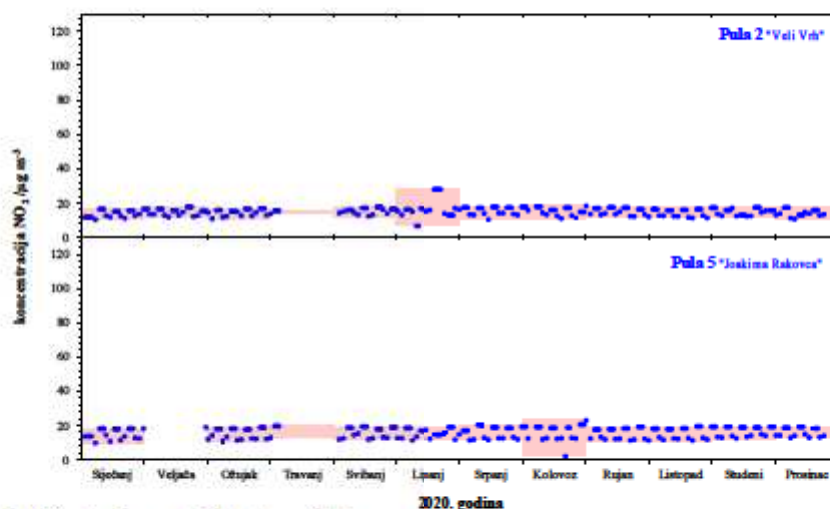
Slika 3. Kretanje srednjih dnevnih koncentracija dušikova dioksida na području Grada Pule u 2020. godini
