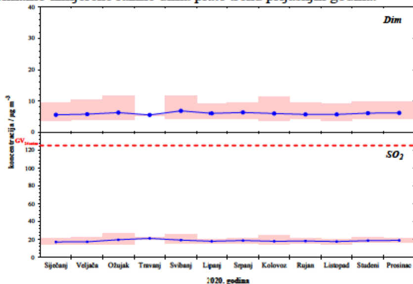
Slika 2. Kretanje srednjih dnevnih koncentracija sumporova dioksida i dima na području Općine Raša u 2020. godini
