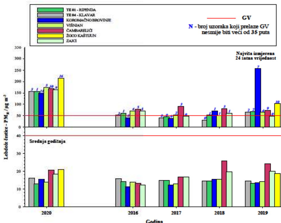
Slika 15. Usporedba rezultata mjerenja koncentracija lebdećih čestica sa kriterijima za vrednovanje kvalitete zraka mjenjenih na automatskim postajama
