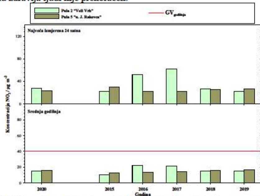
Slika 12. Usporedba rezultata mjerenja dušikova dioksida sa kriterijima za vrednovanje kvalitete zraka na području Grada Pule
