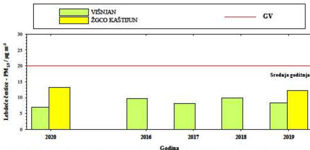
Slika 16. Usporedba rezultata mjerenja koncentracija lebdećih čestica frakcije PM 2,5 sa kriterijima za vrednovanje kvalitete zraka mjerenih na automatskim postajama
