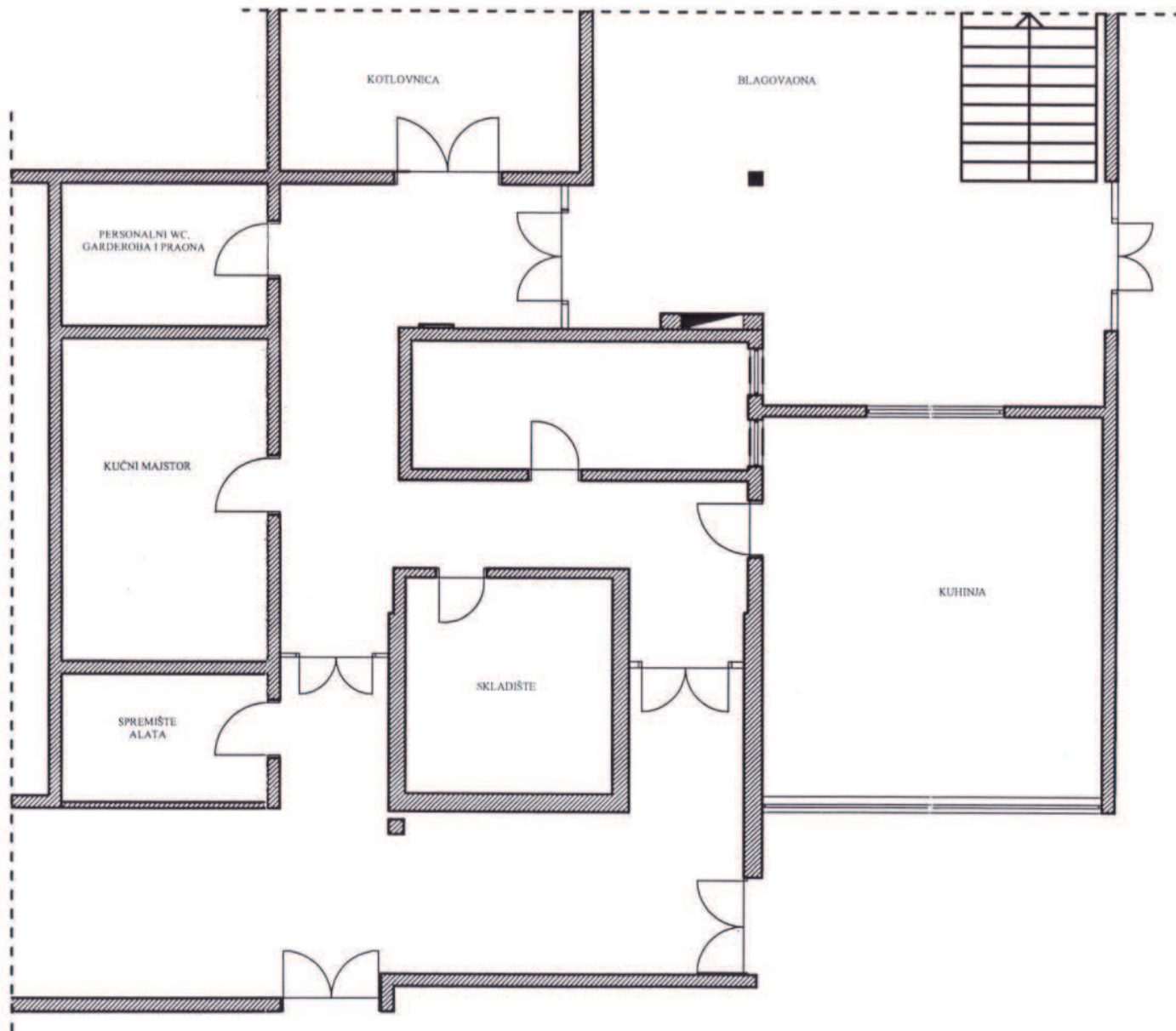
Dječiji vrtić i škola - NOVIGRAD kuhinja - postojeće stanje M 1:100
