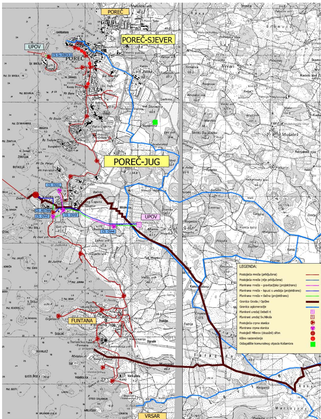
Sl. 1-2 Planirano stanje sustava odvodnje Poreč-jug s izmještanjem uređaja Debeli rt
